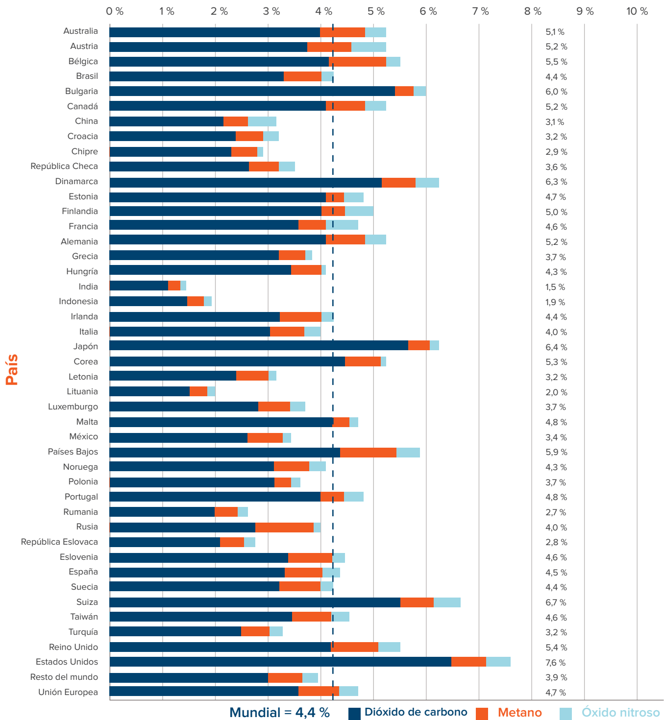
Figura 7: Huella del sector de la salud como porcentaje de las emisiones nacionales de todos los países y regiones abarcados en este estudio
