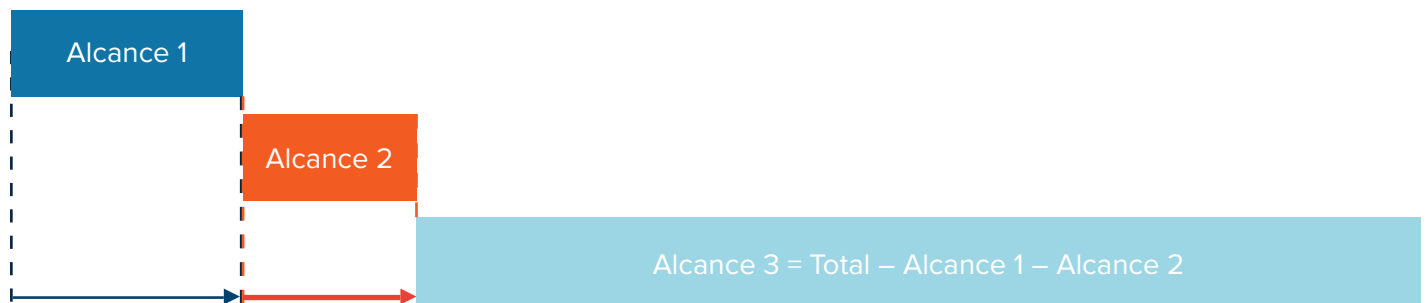
Figura 4: Enfoque adoptado para clasificar las emisiones según las categorías Alcance 1, 2 y 3 del GHGP, a partir del modelo de evaluación de la huella climática del SHA y la WIOD
