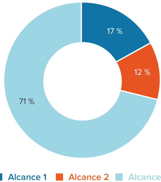
Figura 5: Huella del sector de la salud a nivel global dividida según las categorías de Alcance del GHGP
