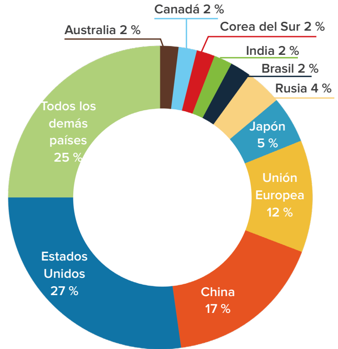
Figura 8: Principales diez emisores más todos los demás países según su porcentaje de la huella global del sector de la salud
