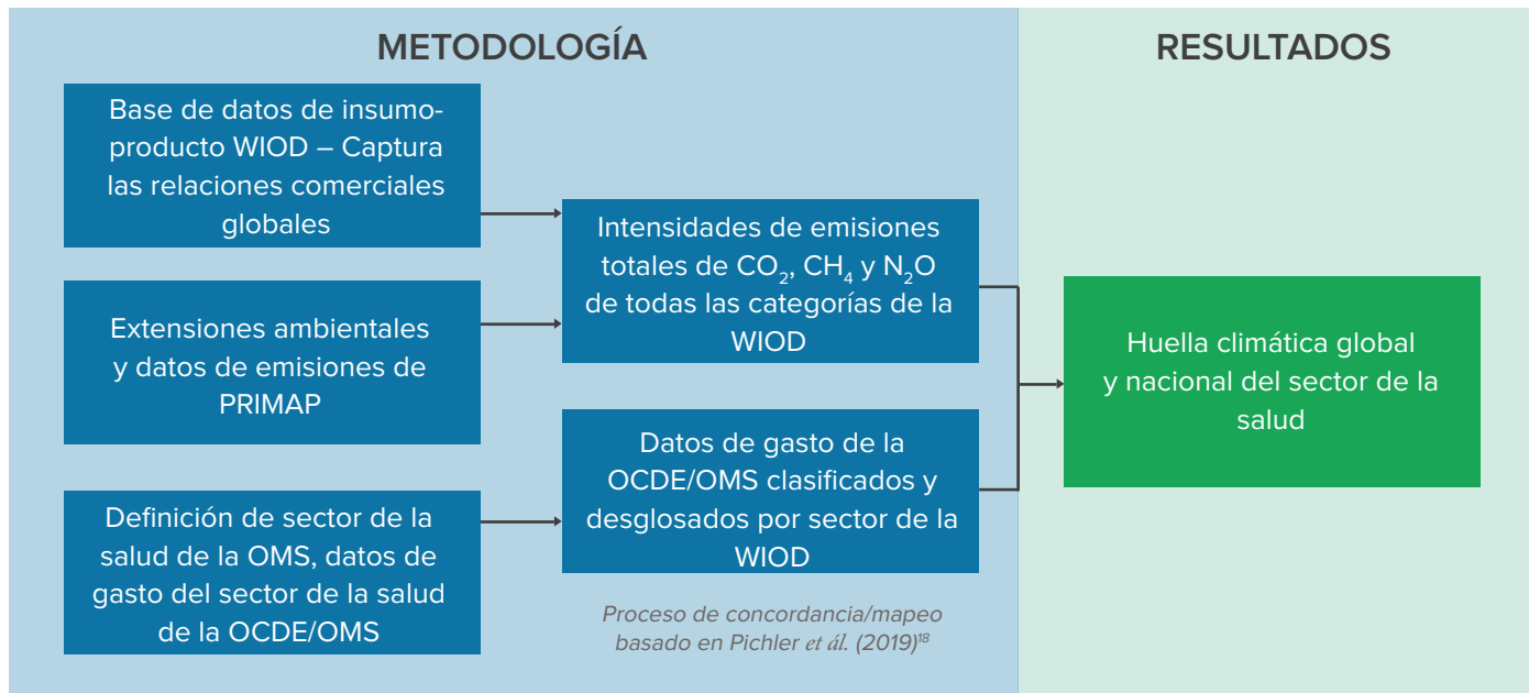
Figura 2: Arquitectura metodológica utilizada por Salud sin Daño para calcular la huella climática del sector de la salud a nivel global
