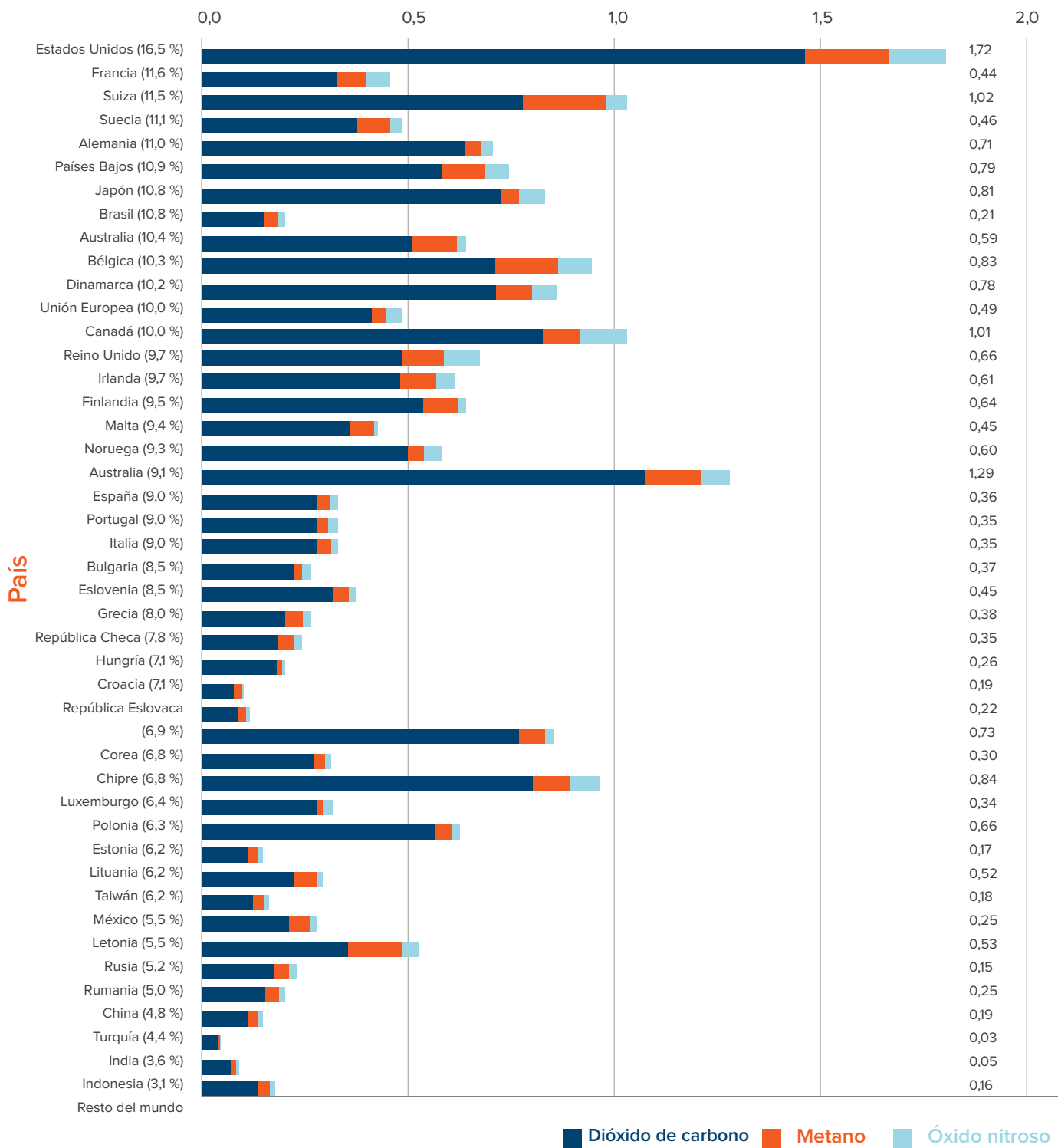
Figura 10: Huella del sector de la salud per cápita ordenada por porcentaje del PBI gastado en salud
