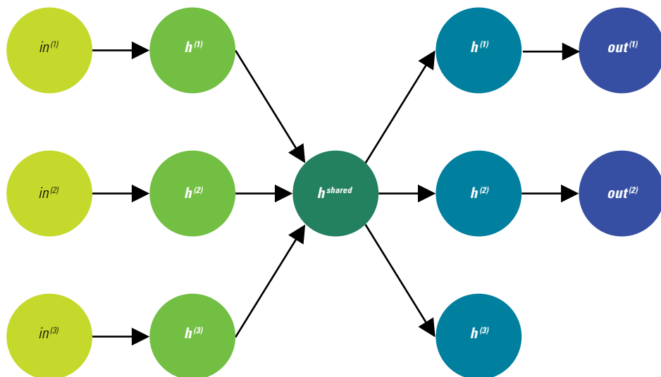
Diagrama VII.2 Arquitectura ilustrativa del aprendizaje multitarea o de transferencia
